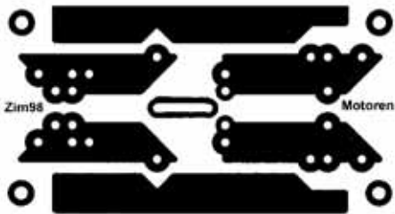
Entstör-Modul für Gleichstrom Elektromotoren
