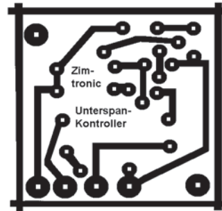
Unterspannungskontrolle
