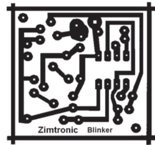
LED Blinkschaltung
