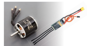
1 x Antriebsset actro-n 35-4-1100 und actrocon 60 A-Regler
