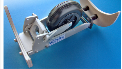
1 × EZKW komplett mit 100-mm-Rad und Bügel, Dämpfungs-Set, Z-Servohalter und gewinkelter Gabelkopf
