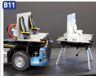
Inneneinrichtungsstecksystem von Servonaut
