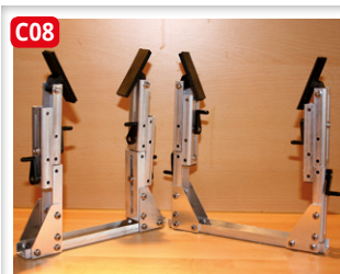
Schiffs-Transportgestell von Tönsfeldt Modellbau-Vertrieb
