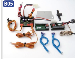
Elektrische Anlage MFL von thicon
