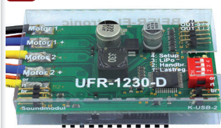
Doppelfahrtregler UFR-1230-D von Beier Electronic
