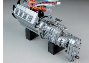
Scale Allradgetriebe 3-Gang von thicon
