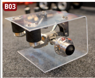
Achsaufhängung mit Luftfederbalg-Attrappen von Comvec
