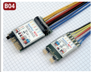
Doppelfahrregler M224 und M211 von Servonaut
