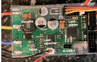
Soundfahrtregler SFR-1 von Beier-Electronic
