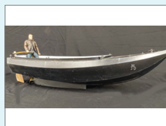
A 12 Vlet Festmacherboot Rumpf von Lextek
