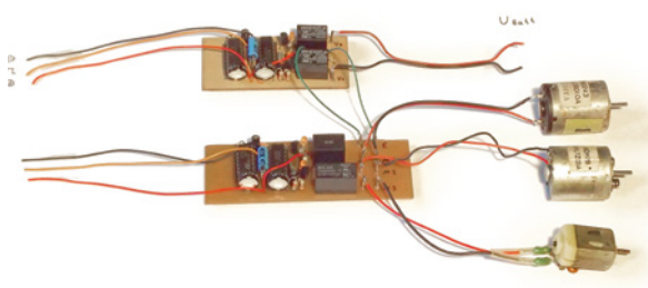
Die Windensteuerung von Wolfram Manske erlaubt das Steuern von drei Winden mit nur zwei Proportional-Kanälen.
