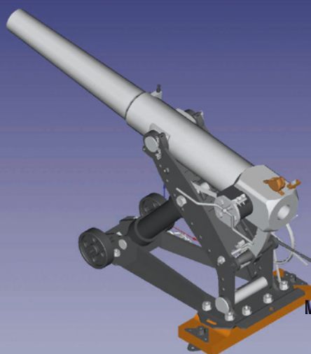
30 Modellbau wird zunehmend digital, wie Dr. Ing. Joachim Pelka am Beispiel eines 8,7-cm-Geschützes der Kaiserlichen Marine zeigt.
