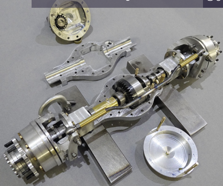
Vorderachse mit vorbildgetreuer Geometrie
